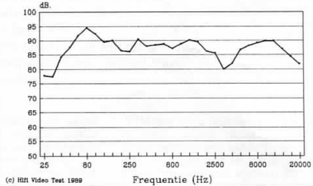
frequentiecurve Translator Impact 50 (huiskamer-simulatie)
