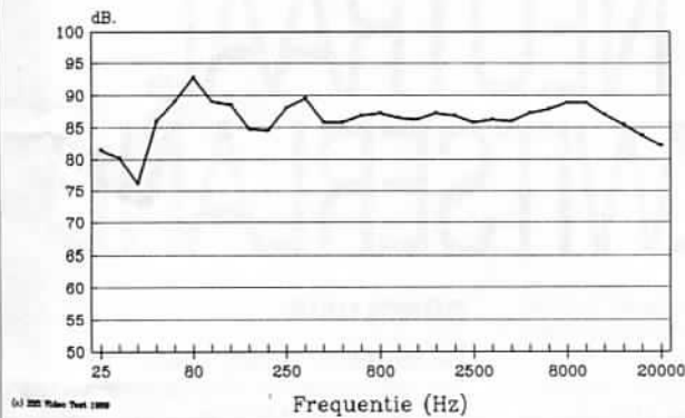
Frequentiecurve Magnat Zero 9 (huiskamer-simulatie)
