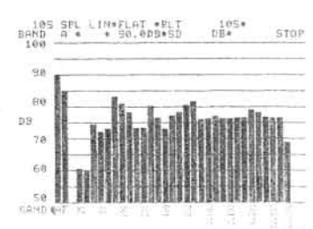
Frequentie-karakteristiek van de Impact 30
